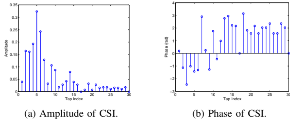
Fig. 4: An example of indoor CSI.
